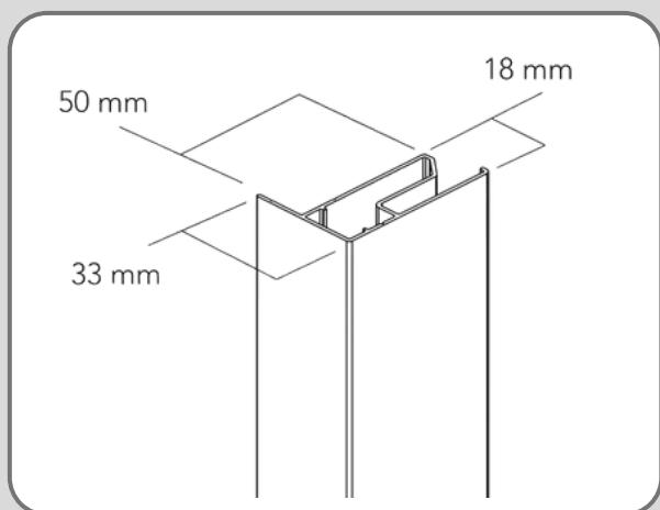
Zijgeleidingsprofiel voor in de dag montage
