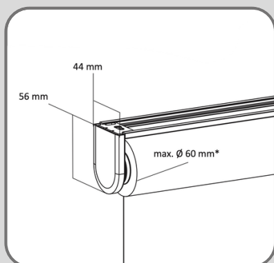
J31 (incl. steun)
