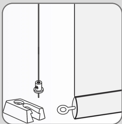
Zijgeleiding met spandraden voor in de dag montage
