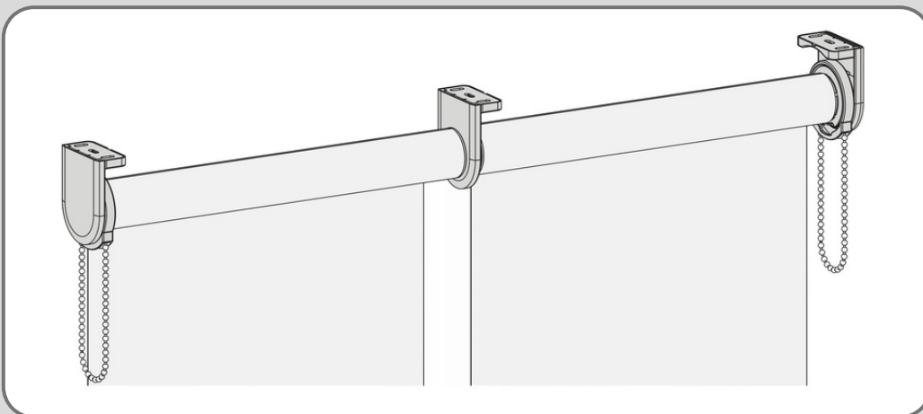
Gekoppeld rolgordijn standaard, dubbele bediening
