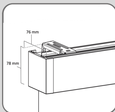
JV32 (incl. steun)
