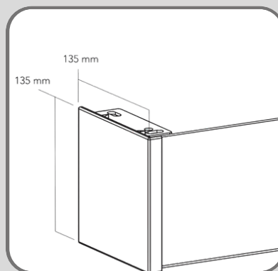
J65 & J85 (incl. steun)
