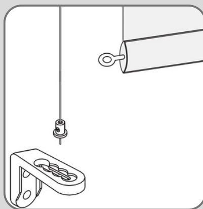
Zijgeleiding met spandraden voor op de dag montage
