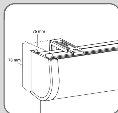
JV34 (incl. steun)
