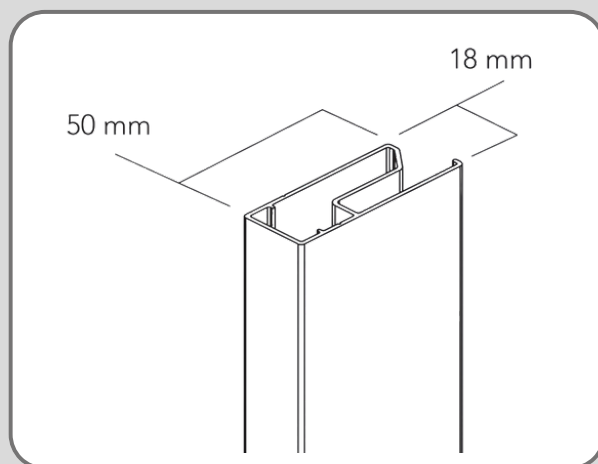
Zijgeleidingsprofiel voor op de dag montage
