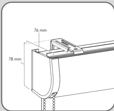
J34 (incl. steun)
