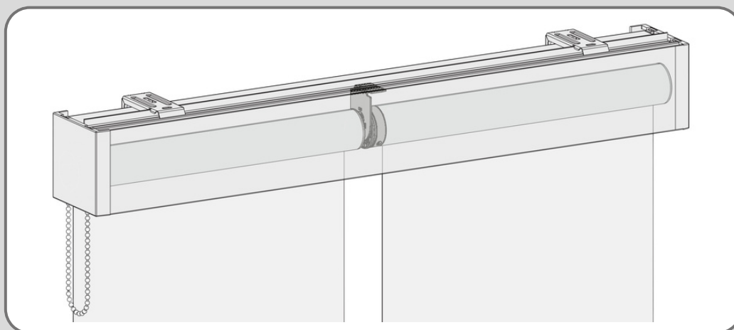
Gekoppeld rolgordijn cassette, enkele bediening
