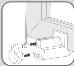
Klemsteun-montage onderzijde
