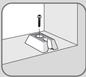
Zijgeleiding in de dag / in het kozijn / in de glaslijst
