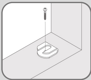
Zijgeleiding in de dag / in het kozijn
