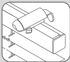
Klemsteun-montage bovenzijde
