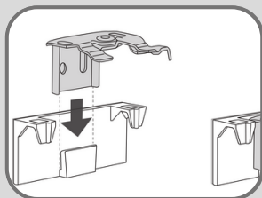
Kleefsteun-montage bovenzijde
