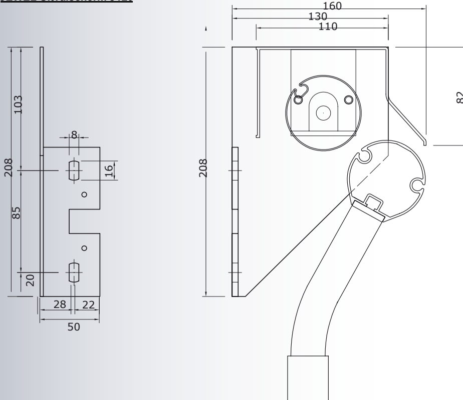
JEWEL Uitvalscherm J120
