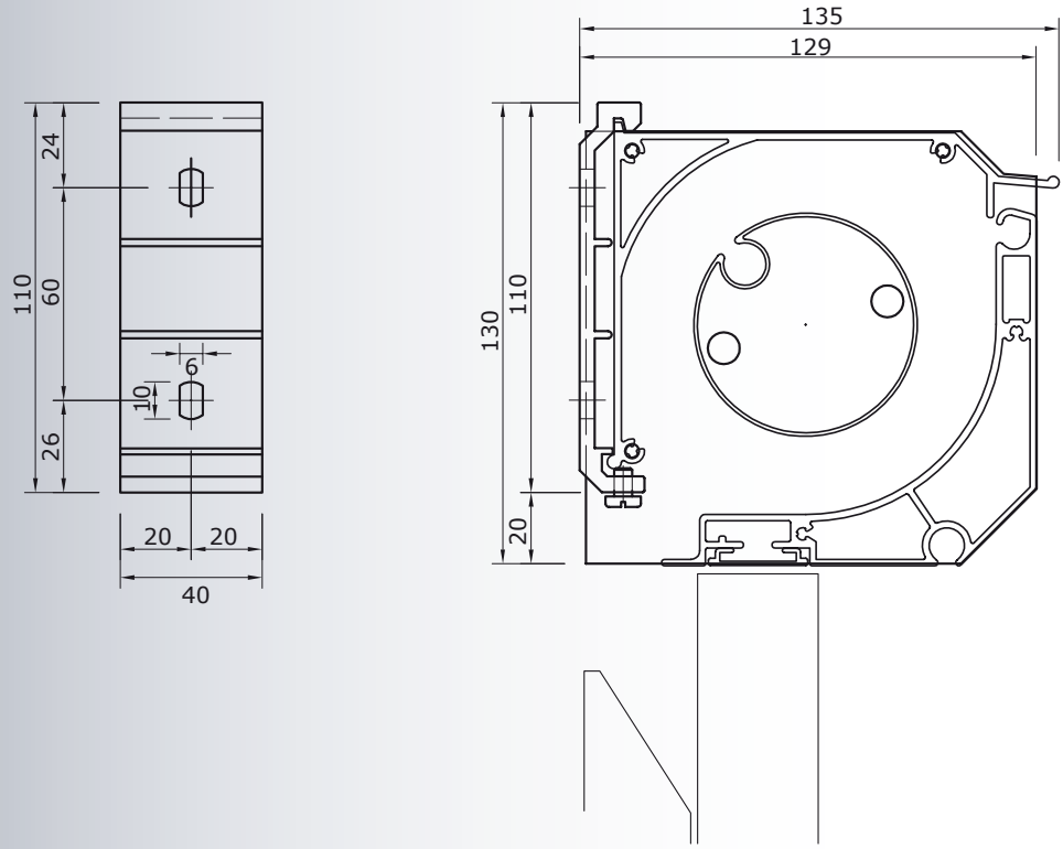
JEWEL Uitvalscherf J170
