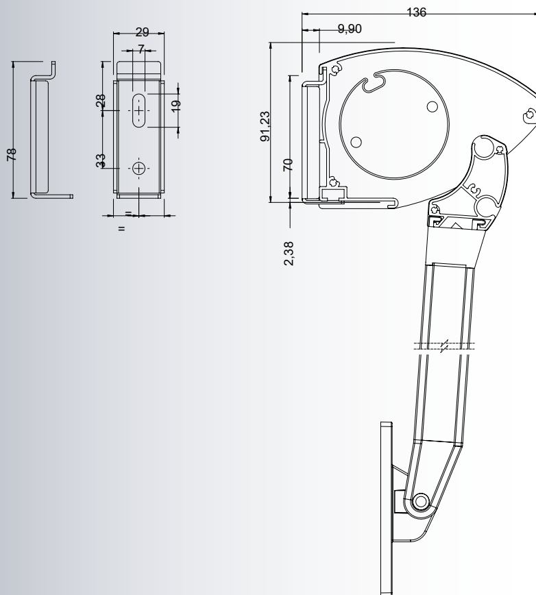
JEWEL Uitvalscherm J124
