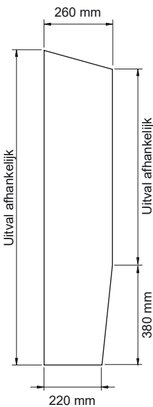
Standaard zijschot
