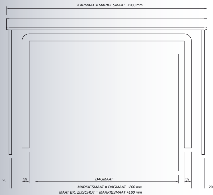
Markies frame hout (Grenen) / bovenkap hout (Red Cedar)
