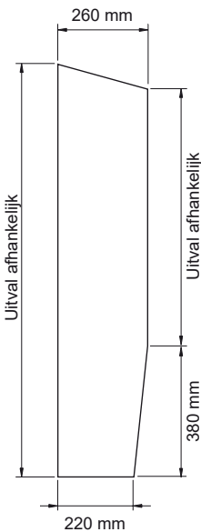
Standaard zijschot
