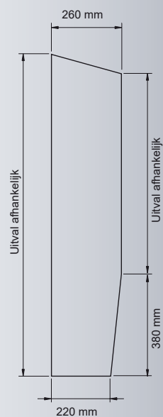
Standaard zijschot
