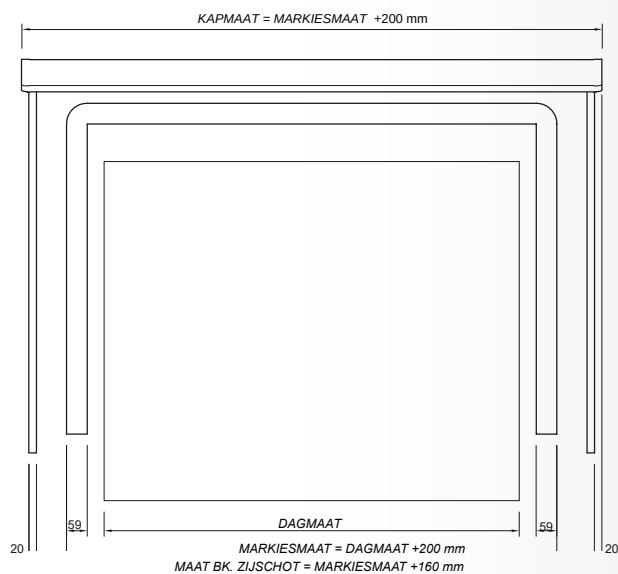
Markies frame hout (Vuren) / bovenkap hout (Red Cedar)
