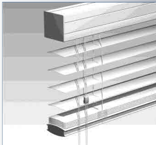
Jaloezie 70 mm.
