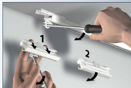
Demontage plafondclip
